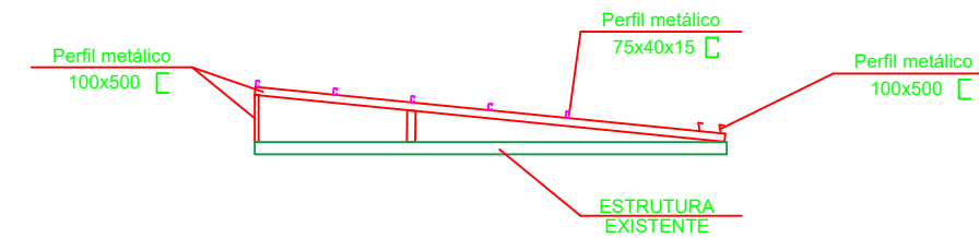
6 ESTRUTURAL - VISTA LATERAL 1/100
