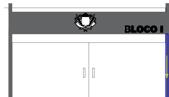
8 PLUVIAL - VISTA FRONTAL 1/100
