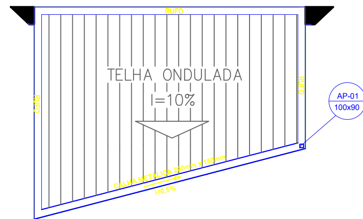
7 PLUVIAL - PLANTA BAXA 1/100
