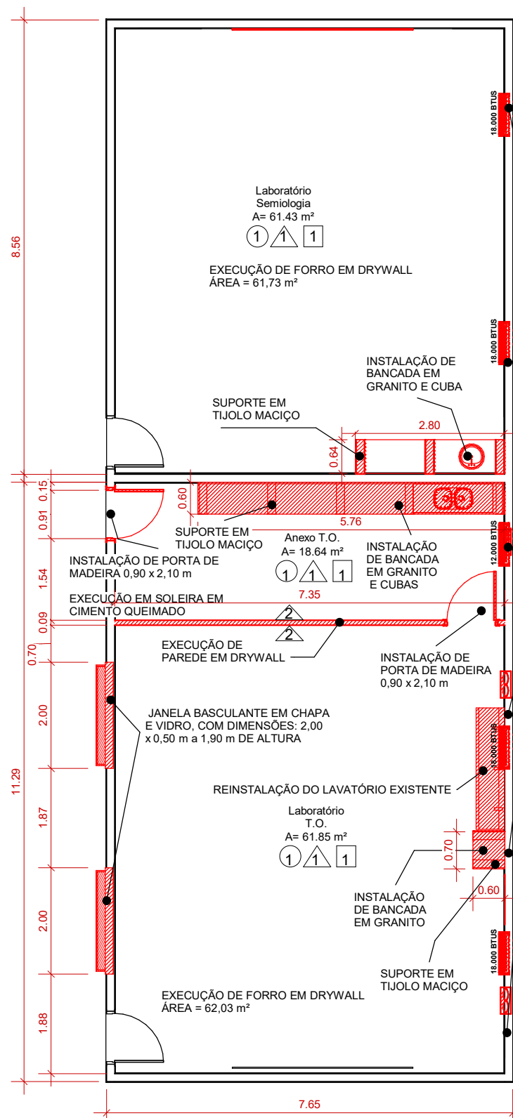
PLANTA BAIXA - EXECUÇÃO
