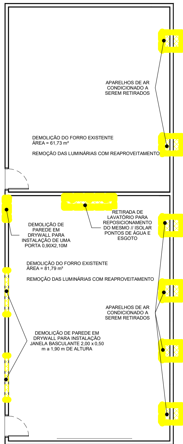
PLANTA BAIXA - DEMOLIÇÃO
