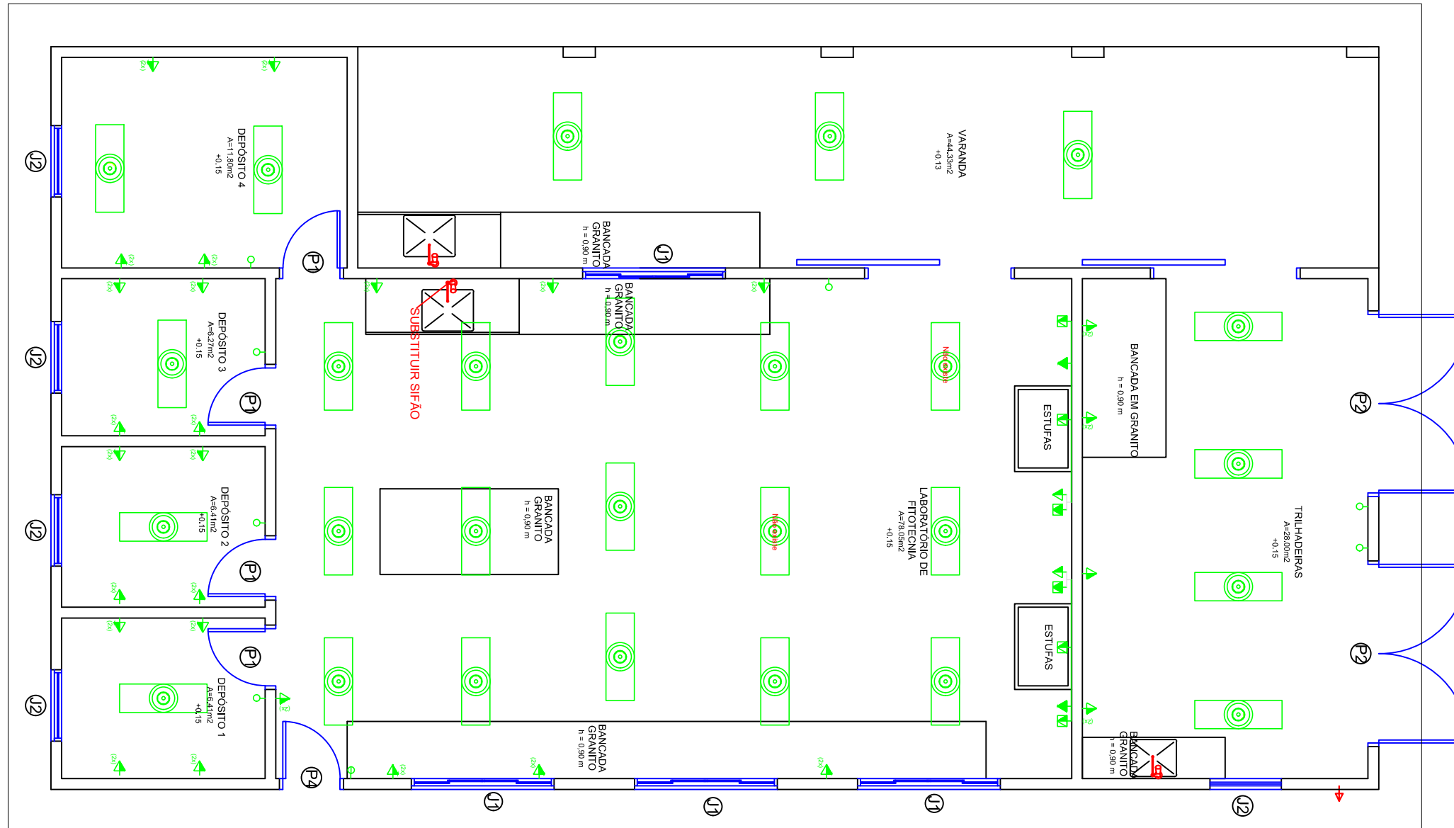
1 Planta Baixa Reforma - Elétrica e Hidráulica 1:75
