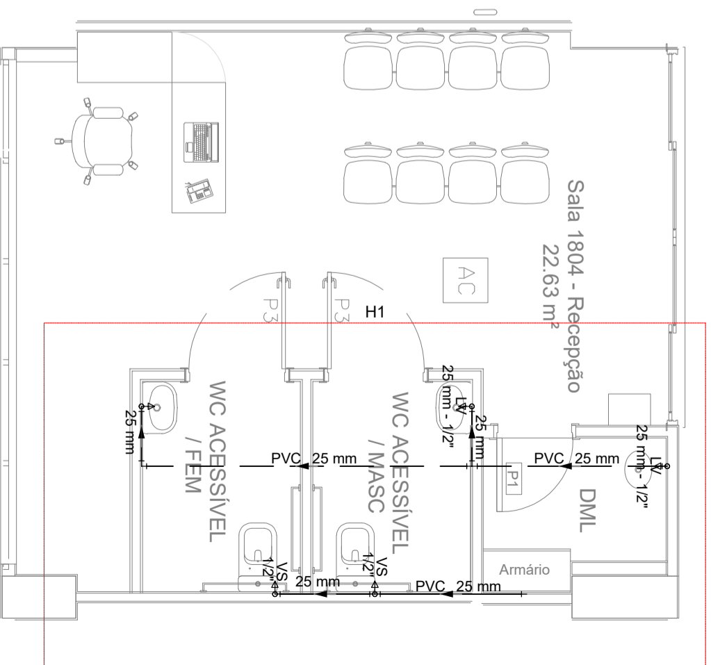
PROJETO DE INSTALAÇÕES HIDRÁULICAS ESC. 1:50
