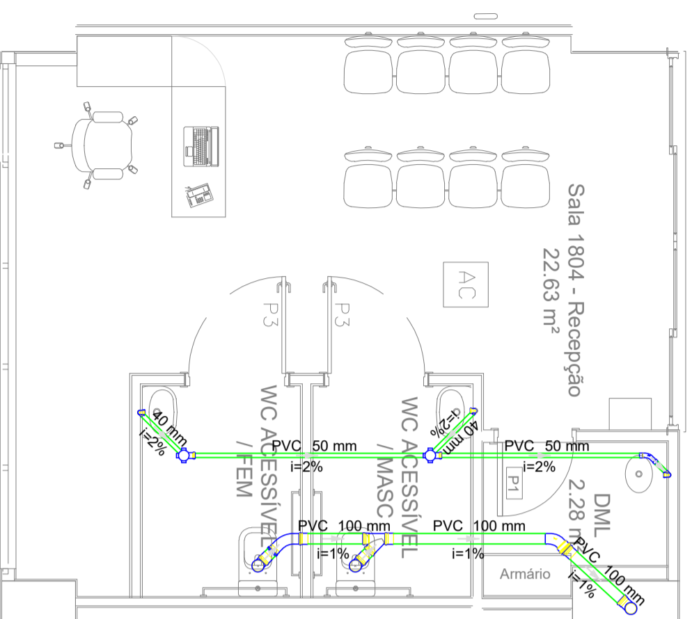
PROJETO DE INSTALAÇÕES SANITÁRIAS ESC. 1:50
