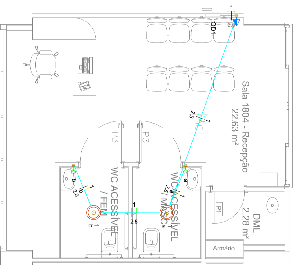
PROJETO DE INSTALAÇÕES ELÉTRICAS ESC. 1:50
