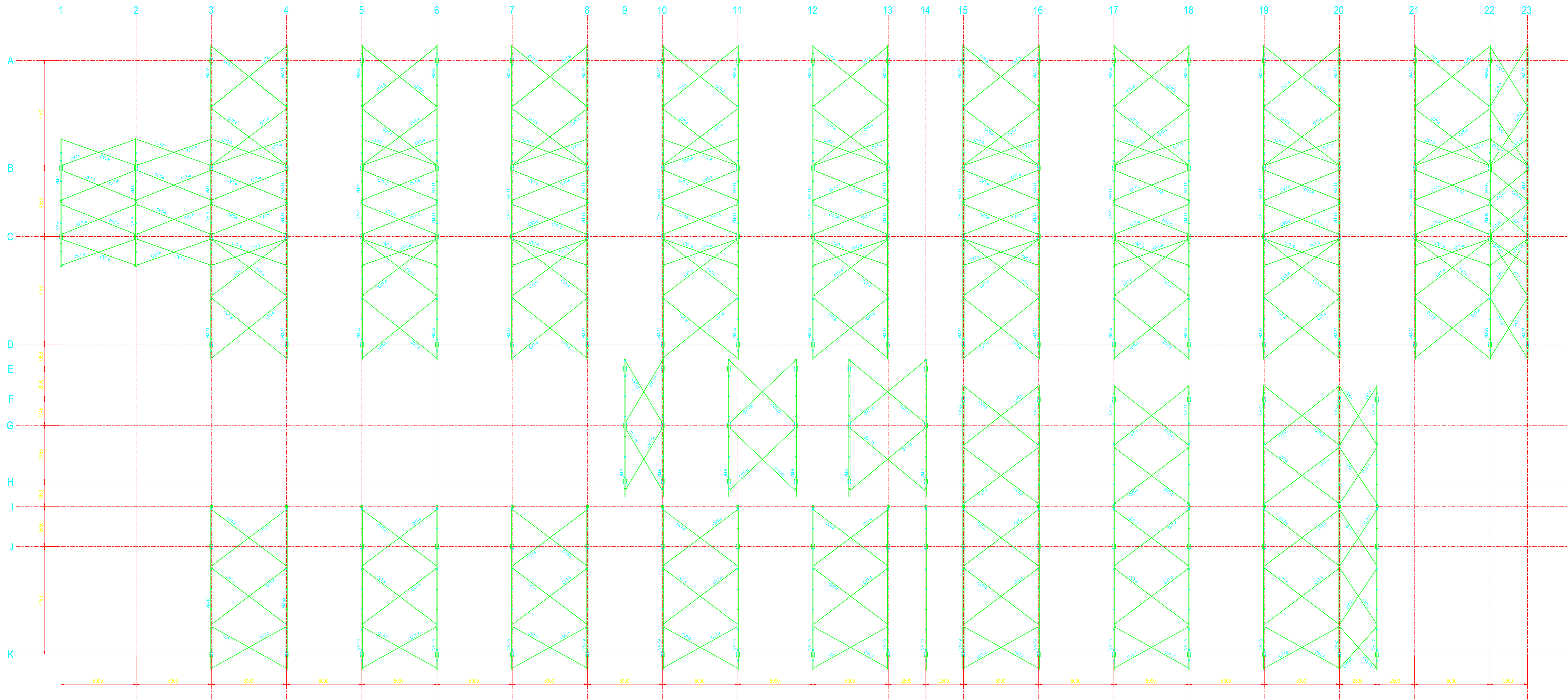
PLANTA DA COBERTURA - VIGAS E CONTRAVENTAMENTOS
