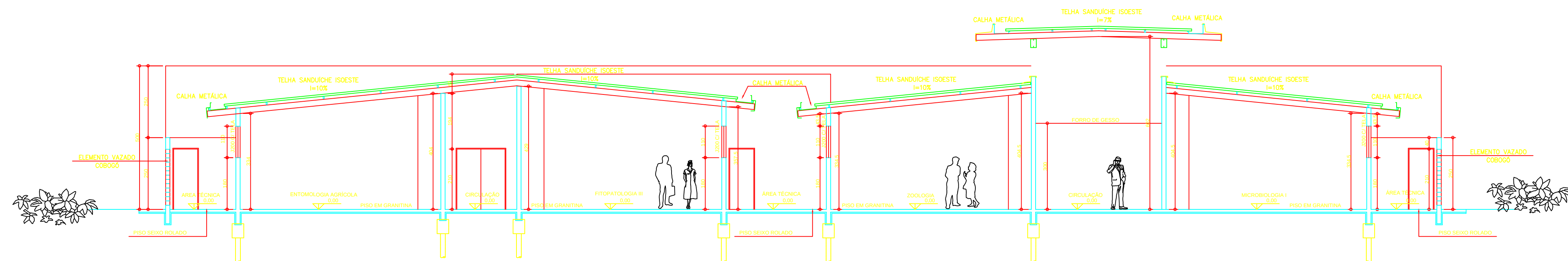
2 CORTE TRANSVERSAL AA' Esc. 1:100
