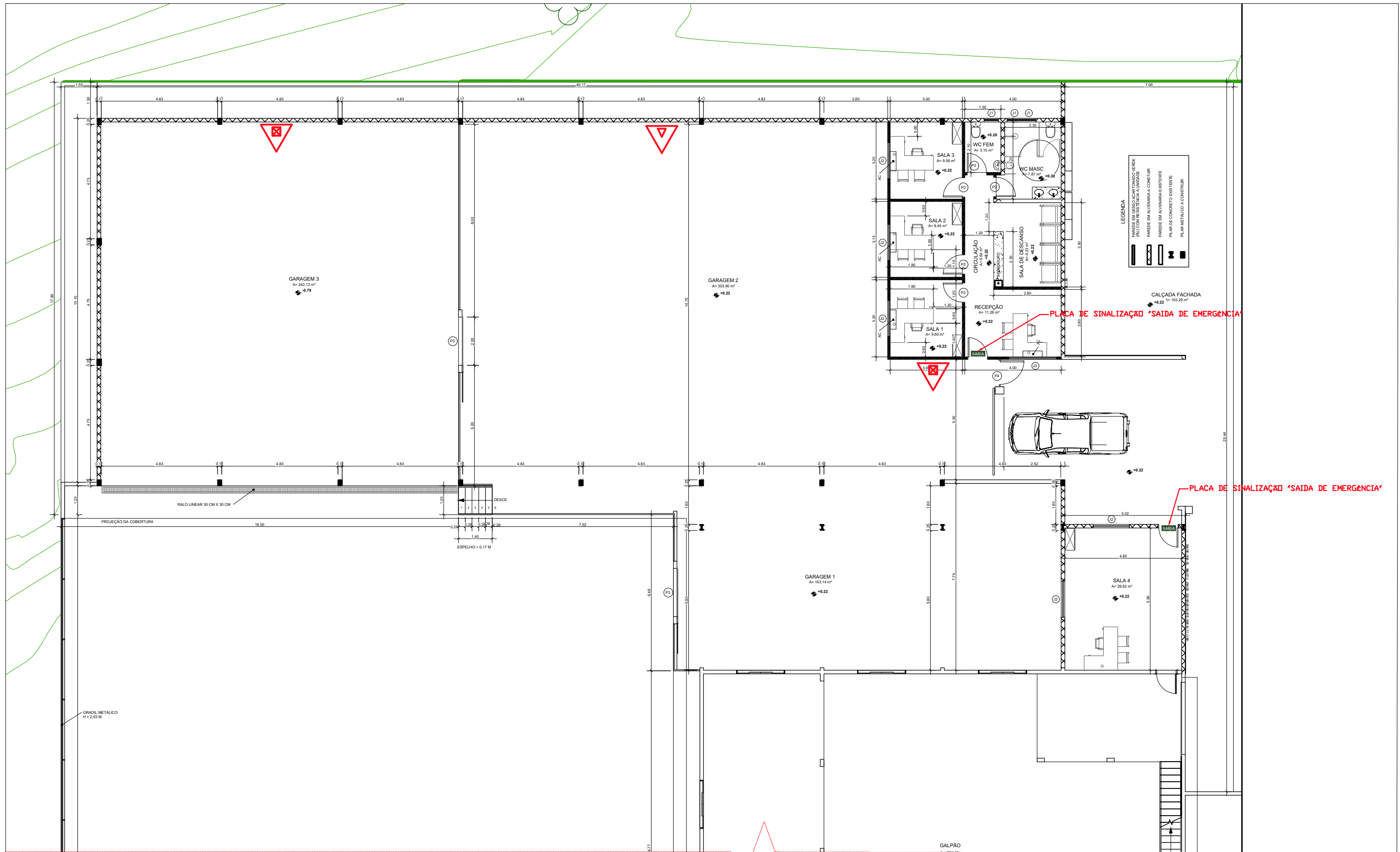
① PLANTA BAIXA - PROJETO DE PREVENÇÃO E COMBATE E À INCÊNDIO Esc. 1:150
