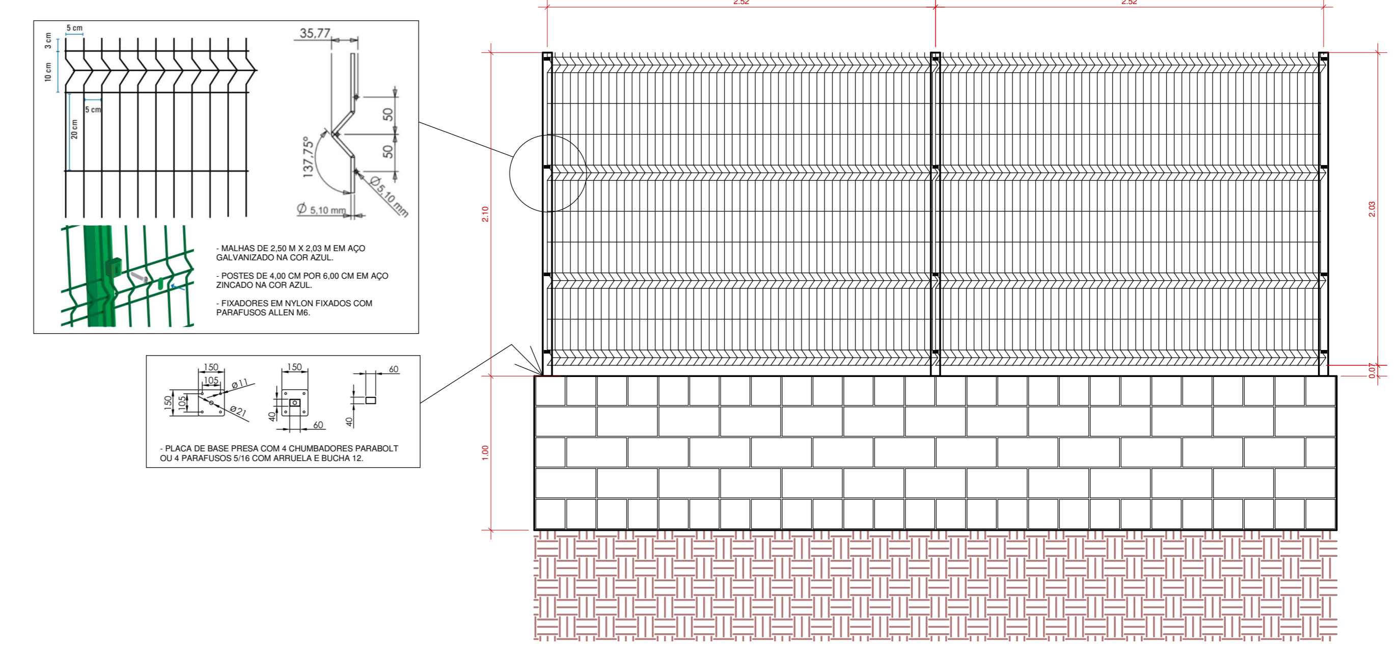
DETALHE GRADIL ESCALA: 1 : 25
