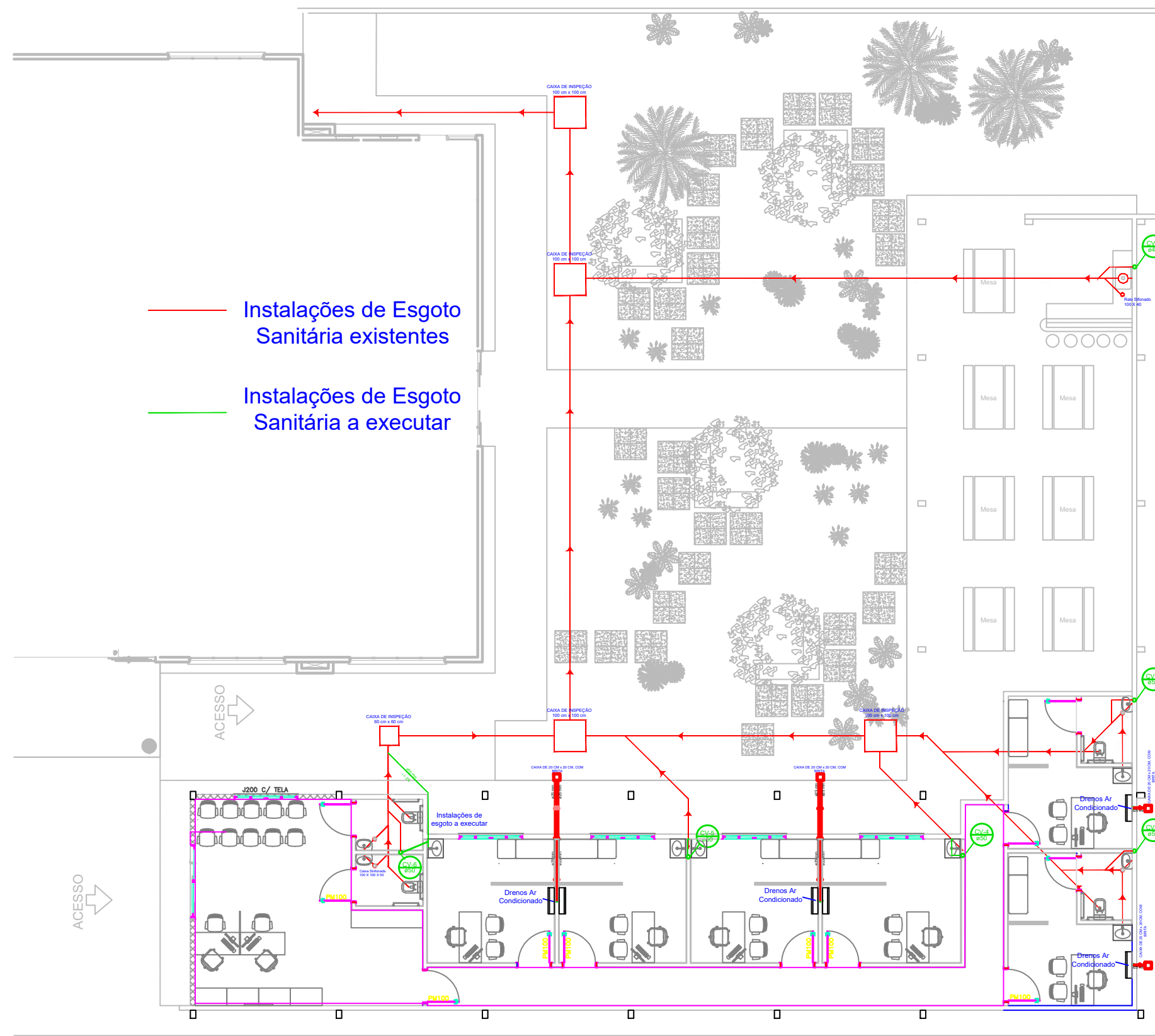
PLANTA BAIXA PROJETO ESGOTO escala 1:150
