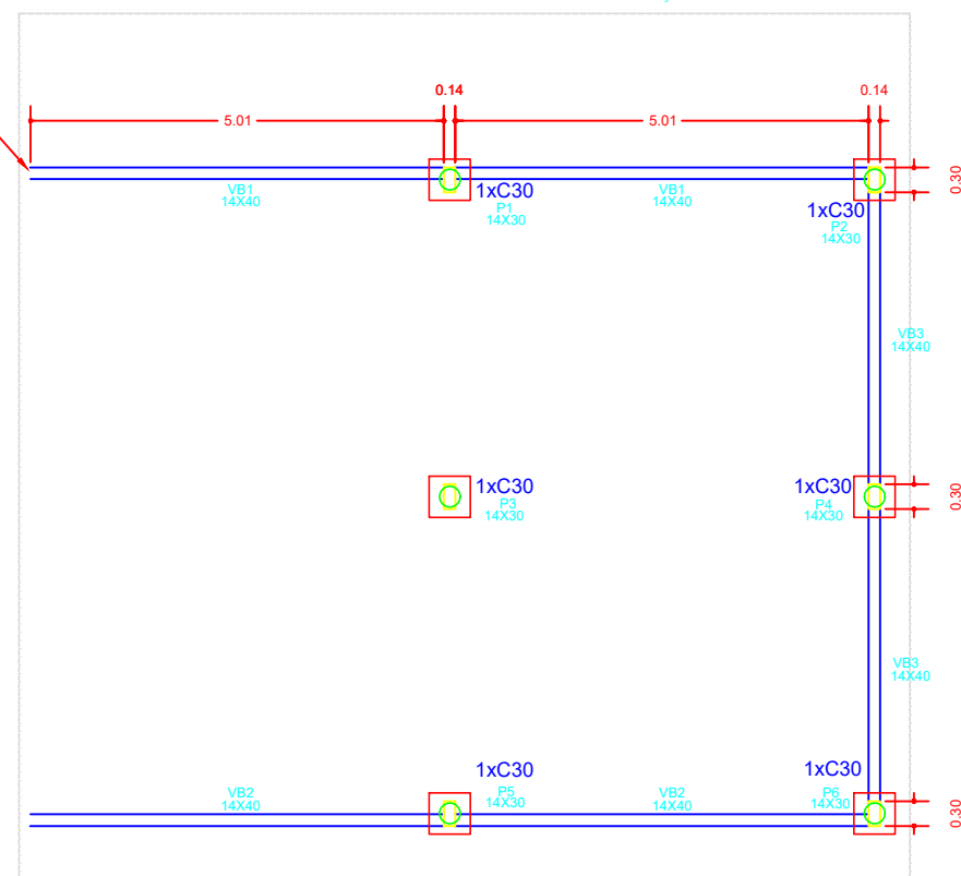
PLANTA - FORMA BALDRAME ESC.: 1:50
