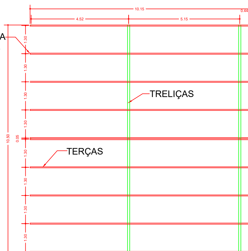
PLANTA - ESTRUTURA METÁLICA ESC.: 1:50
