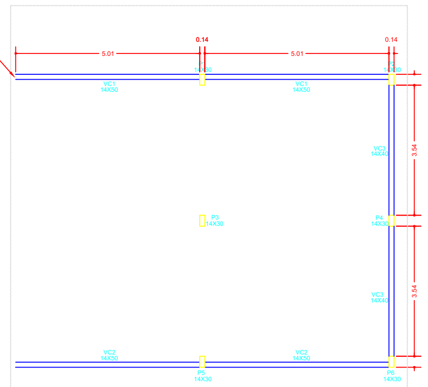
PLANTA - FORMA VIGAS COBERTURA ESC.: 1:50
