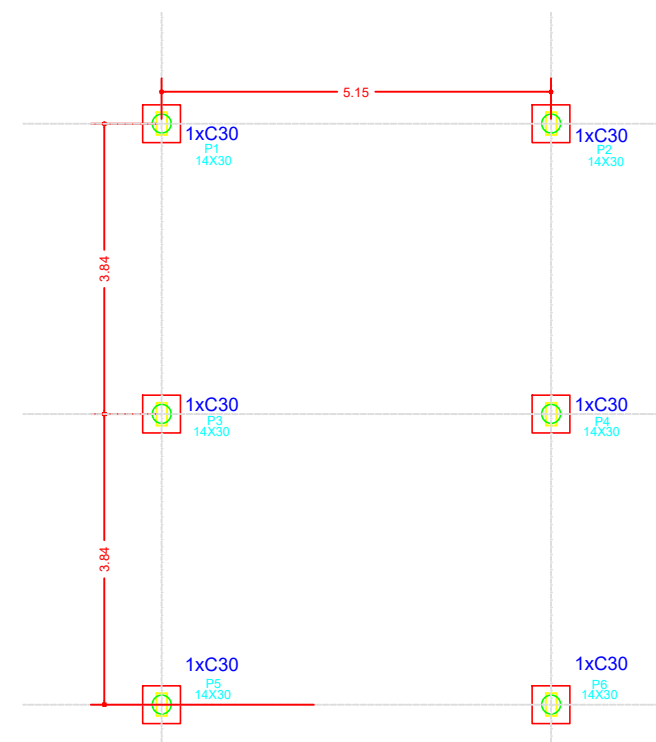
PLANTA - LOCAÇÃO DAS FUNDAÇÕES ESC.: 1:50
